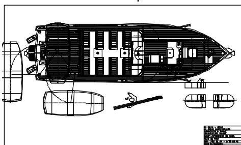
Plan de pont
