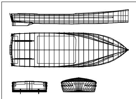
Plan des formes
